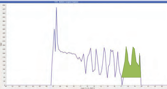
CURVA CONSUMO CALEFACCIÓN SEMANA TIPO ENE
