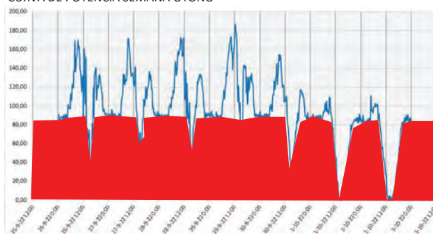
CURVA DE POTENCIA SEMANA OTOÑO
