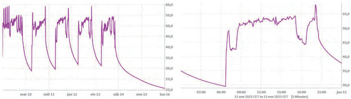
EVOLUCIÓN DE LA TEMPERATURA DE IMPULSIÓN DE AGUA EN COLECTOR. AULARIO IndUva. ENERO 2023
