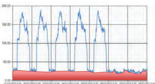
CURVA POTENCIA SEMANA INVIERNO 2021
