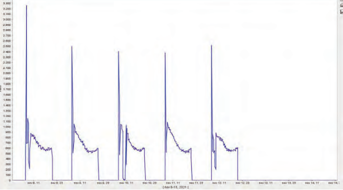
CURVA DE CONSUMO CALEFACCIÓN SEMANA TIPO NOVIEMBRE
