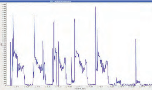
CURVA CONSUMO CALEFACCIÓN SEMANA TIPO NOV
