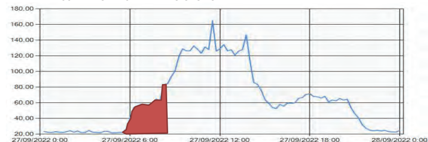
CURVA POTENCIA DÍA TIPO OTOÑO
