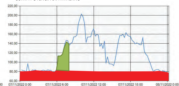
CURVA POTENCIA DÍA INVIERNO
