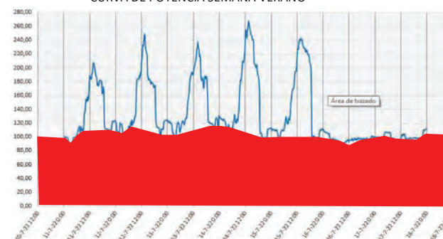
CURVA DE POTENCIA SEMANA VERANO
