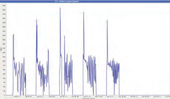
CURVA CONSUMO CALEFACCIÓN DÍA TIPO NOV
