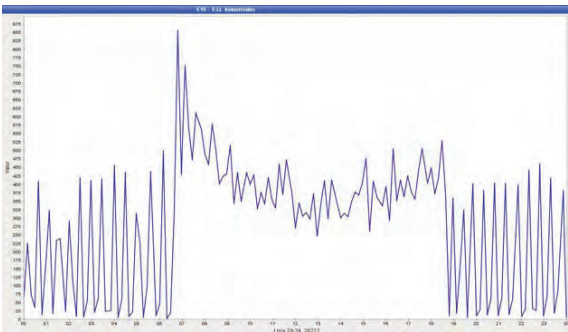
CURVA CONSUMO CALEFACCIÓN DÍA TIPO NOV. CAUCE
