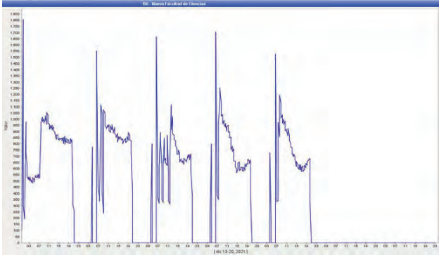
CURVA DE CONSUMO CALEFACCIÓN DÍA TIPO ENERO
