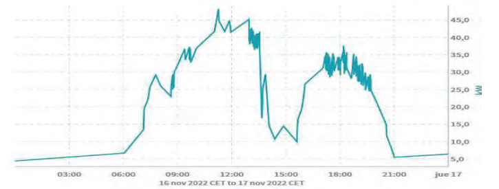
CURVA DE POTENCIA DÍA TIPO NOV. AULARIO IndUVa
