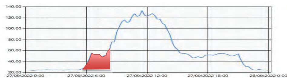
CURVA POTENCIA DÍA TIPO OTOÑO
