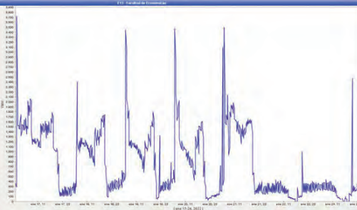
CURVA CONSUMO CALEFACCIÓN SEMANA TIPO ENE
