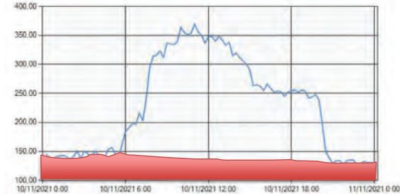
CURVA POTENCIA DÍA INVIERNO 2021
