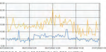
EDIFICIO E. CURVA DE POTENCIA DÍA TIPO INVIERNO
