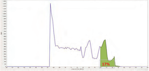
CURVA CONSUMO CALEFACCIÓN DÍA TIPO ENE
