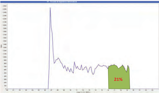
CURVA CONSUMO CALEFACCIÓN DÍA TIPO ENE
